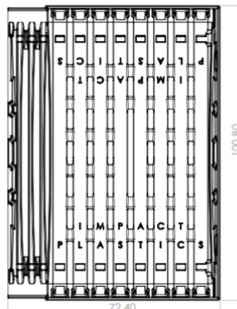
Le couvercle est niché sur une des trois cotés formés dans la pièce. Ceci permet de couvrir une fourchette de 12' à 22'
